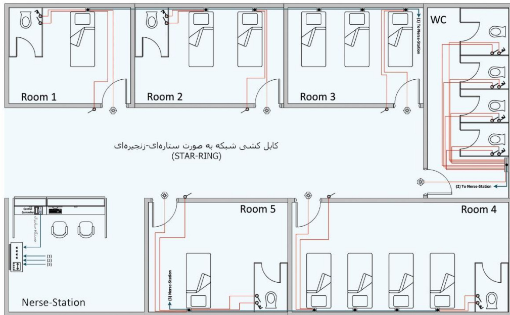
شماتیک یک بخش بستری نمونه و کابل کشی مربوط به سیستم احضار پرستار آرنیکا
